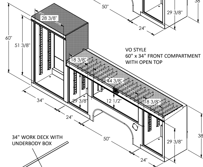
VO STYLE OPEN TOP
